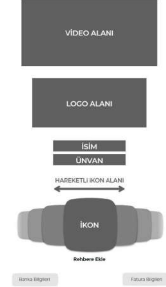
16.1 Grafikselsel Kullanıcı Arayüzü (Dijital Kartvizit için)
